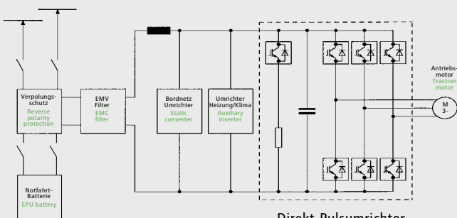
Direkt-Pulsumrichter mit Bremssteller Traction inverter with brake chopper
